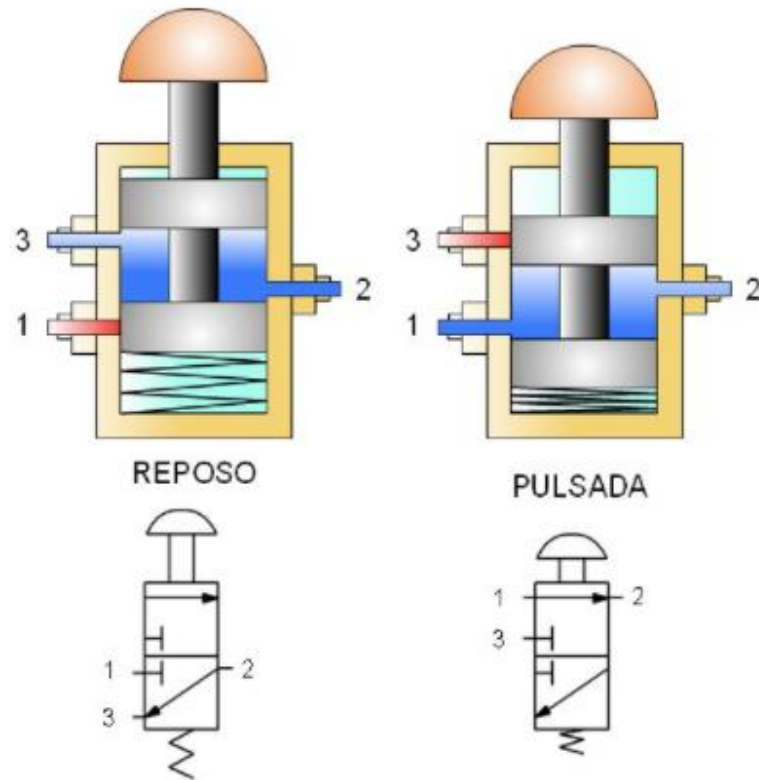
Válvula 3/2 normalmente cerrada
